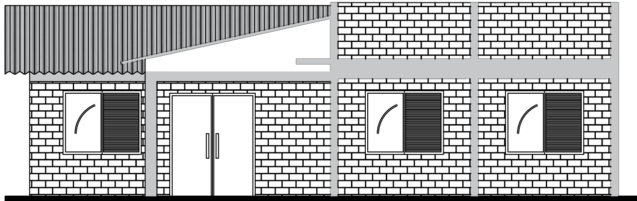
1 FACHADA Escala: 1:75
